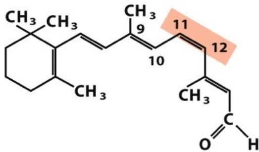
11-cis-Retinal
