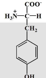
Tyrosine
