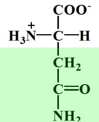
Asparagine
