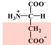
Aspartate
